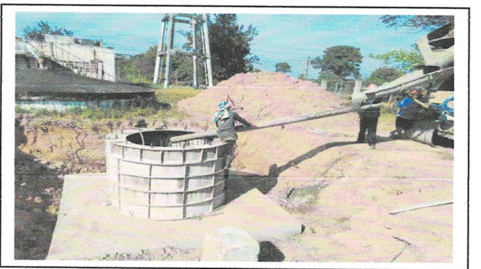
๓๖. โครงการเพิ่มประสิทธิภาพการผลิตน้ำประปาสะอาด เพื่อเก็บกักเป็นน้ำต้นทุน สำหรับการอุปโภค-บริโภค ในช่วงฤดูแล้ง บ้านอาโพน หมู่ที่ ๑ ตำบลอาโพน อำเภอบัวเขต จังหวัดสุรินทร์
